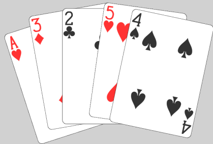
GoofSpiel
